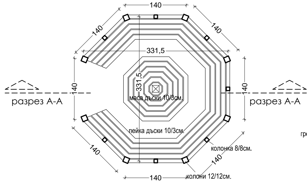
ПЛАН М1:50
