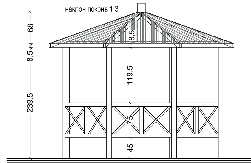
ИЗГЛЕД М1:50
