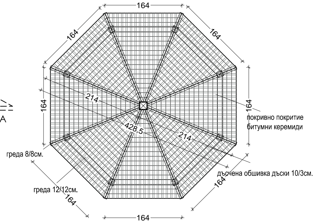
ПЛАН ПОКРИВ М1:50
